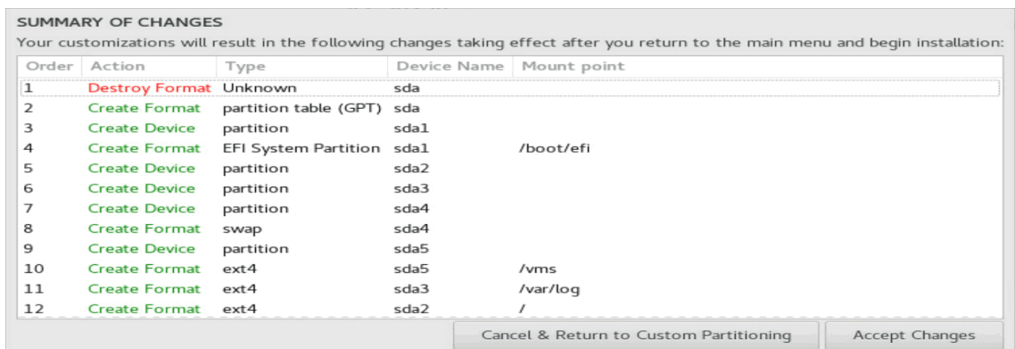
图4-8 确认对话框
