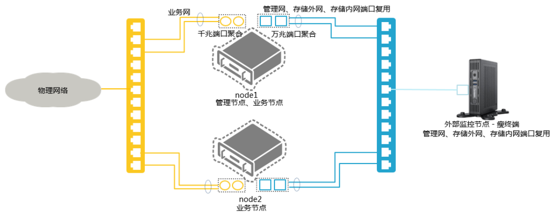
图3-6 两节点方案逻辑网络拓扑（虚拟机）
