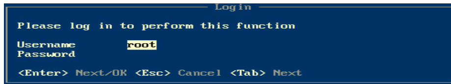
图5-7 Login 对话框
