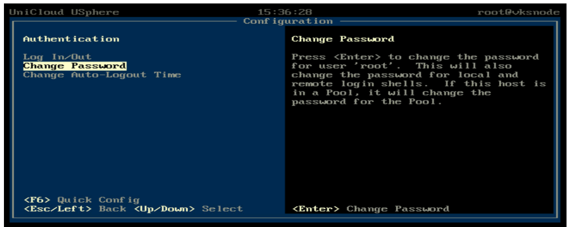
图5-6 Authentication 页面
