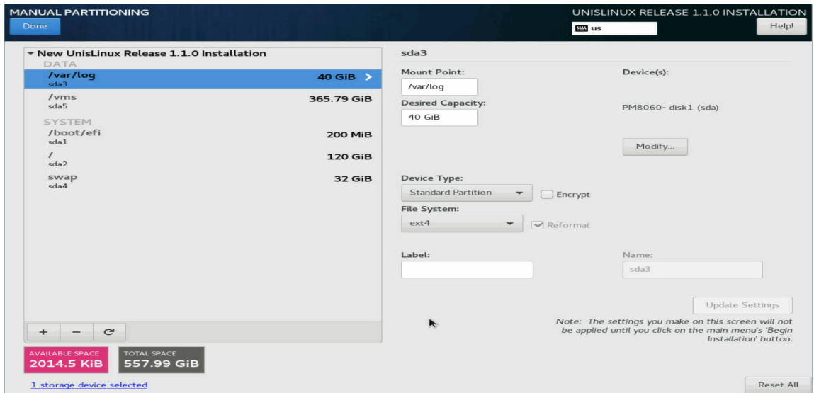
图4-7 分区完成
