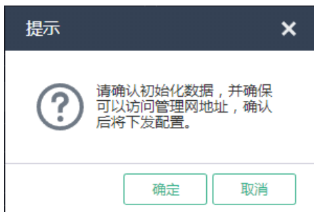
图5-14 提示对话框
