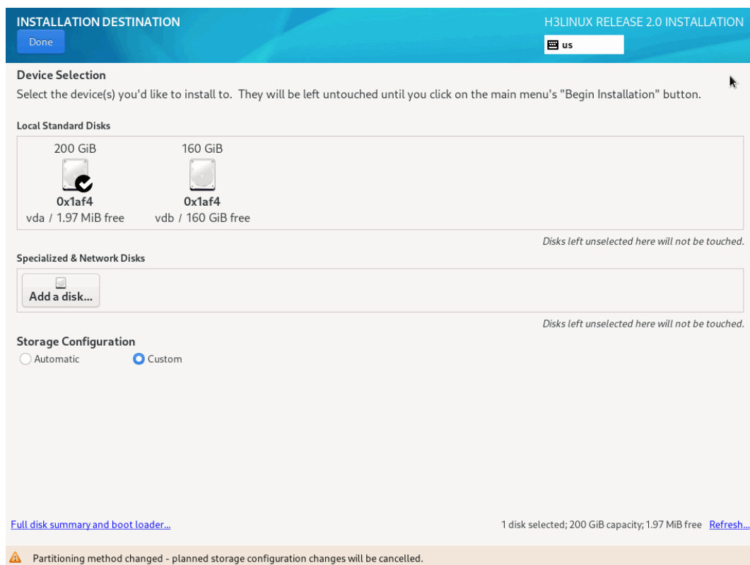
图4-13 选择系统盘-手动分区
