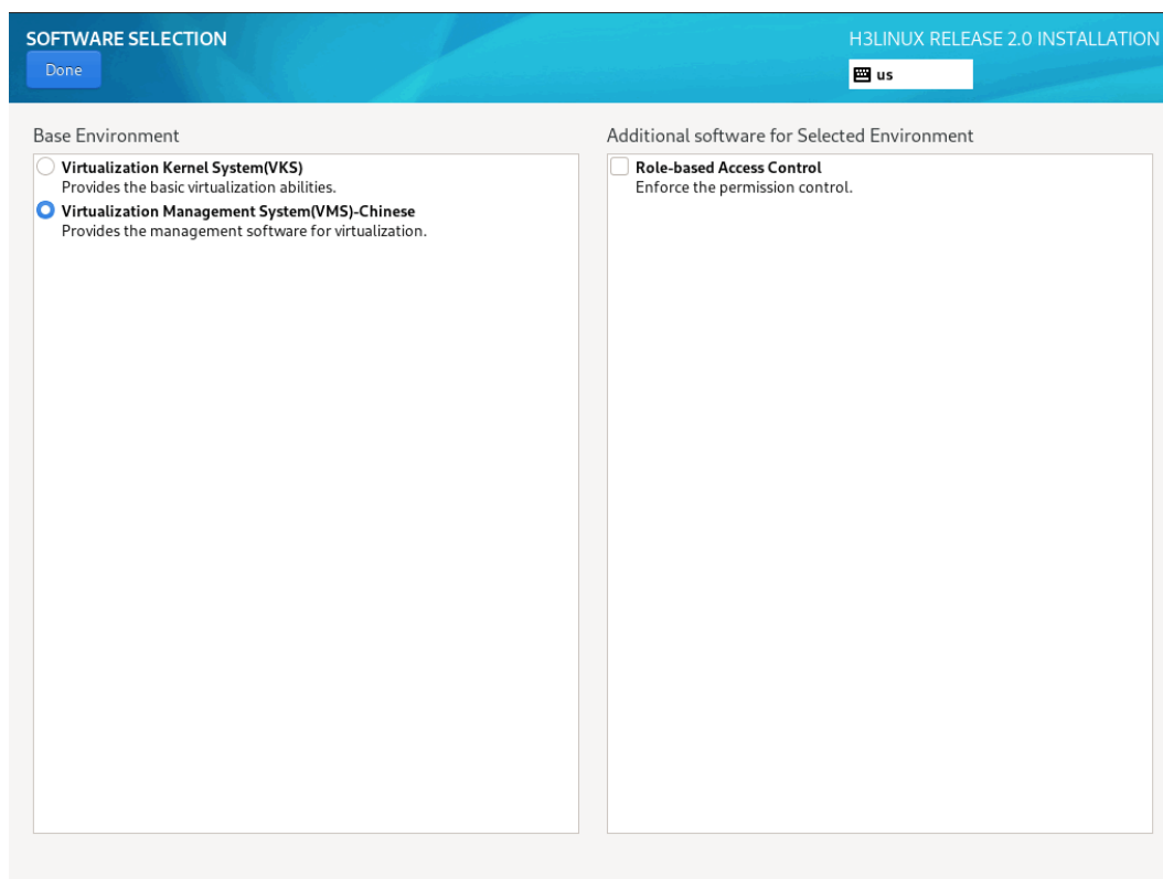
图4-20 根据服务器类型选择安装 Usphere 组件
