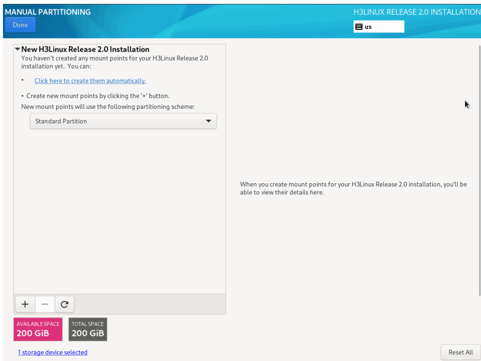
图4-14 手动分区页面
