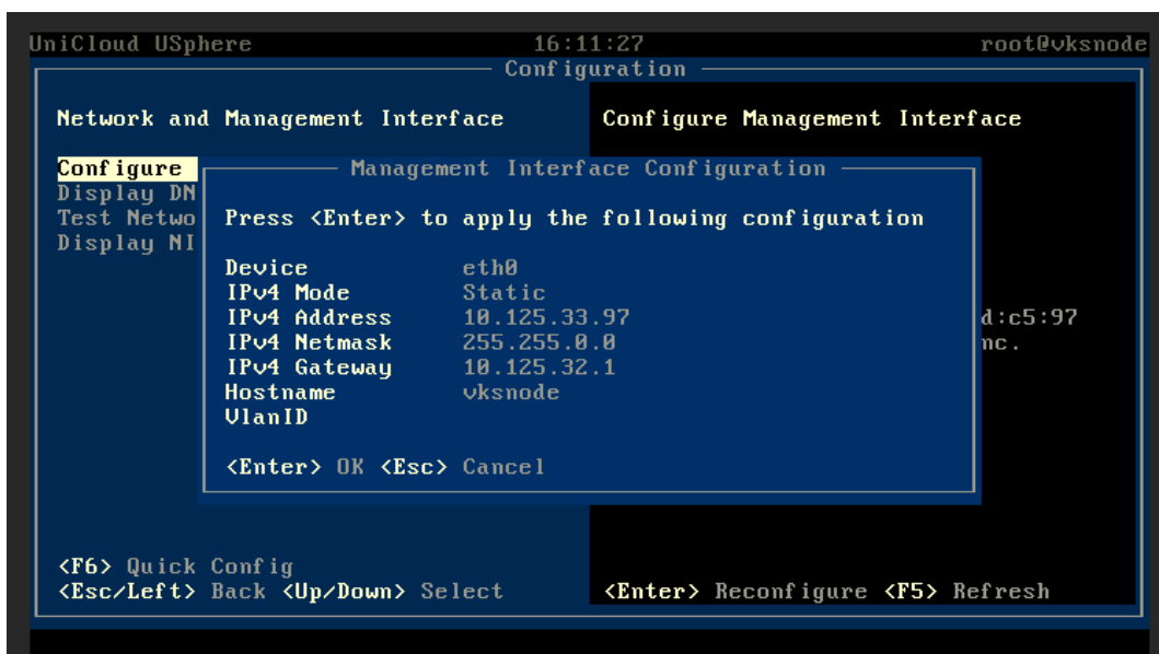
图4-29 设置静态 IP 页面
