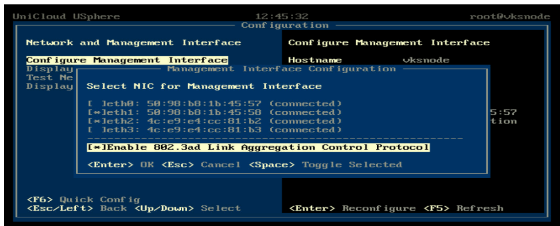
图4-30 配置链路聚合
