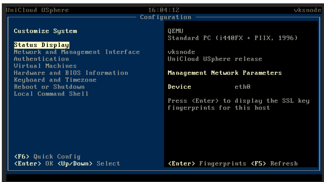
图4-25 参数配置页面
