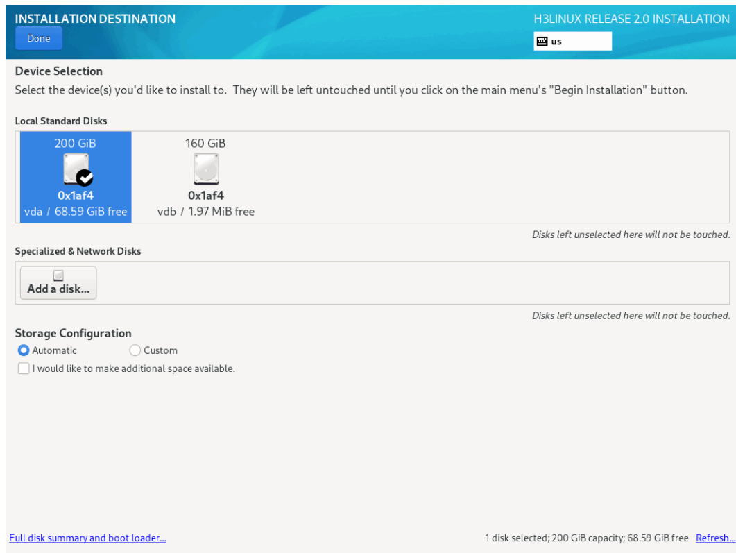
图4-11 选择系统盘-自动分区
