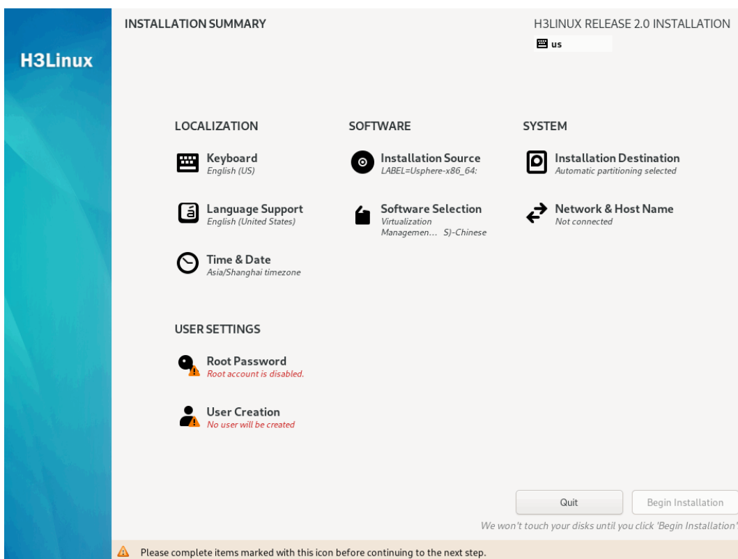
图4-5 系统安装页面
