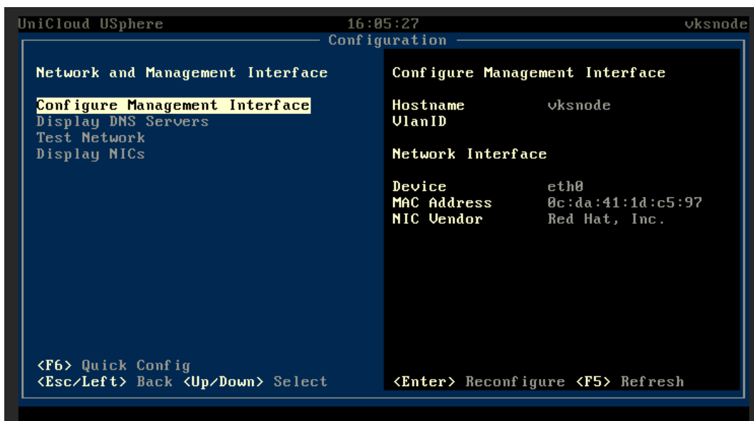
图4-26 Configure Management Interface 页面
