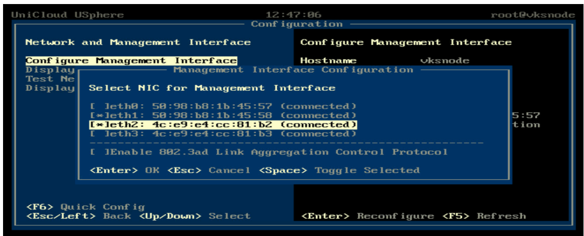
图4-32 配置链路聚合
