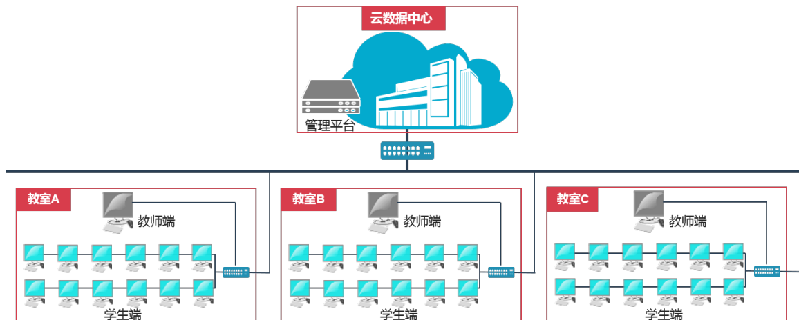
图1-1 组件关系图
