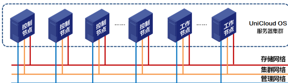
图7-1 组网方案
