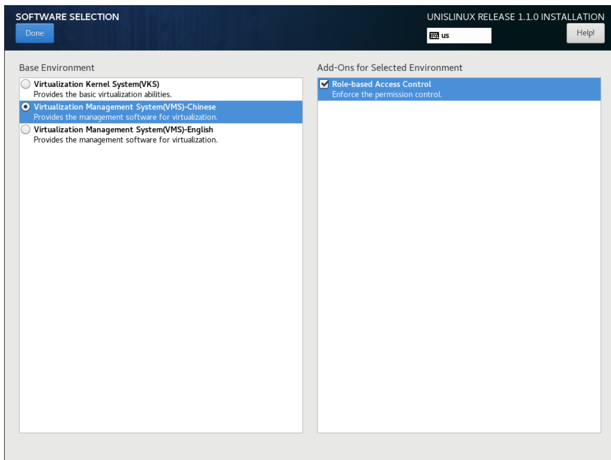
图4-22 根据服务器类型选择安装 Usphere 组件
