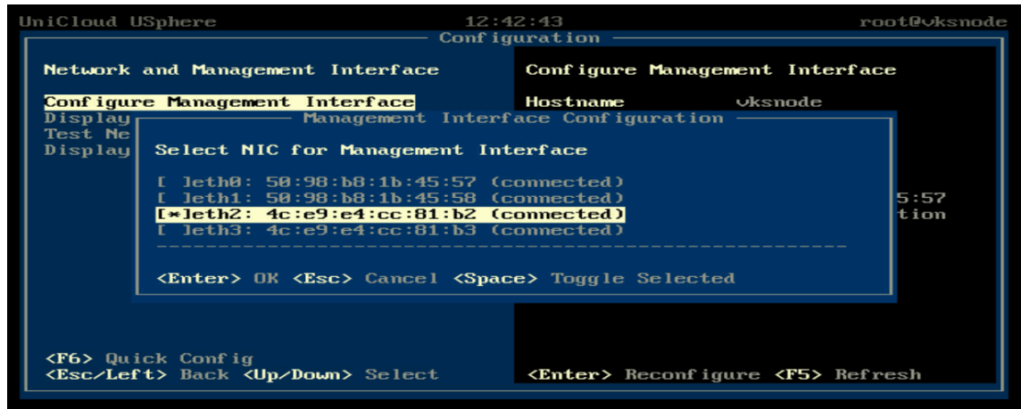
图4-28 选择管理网网卡页面
