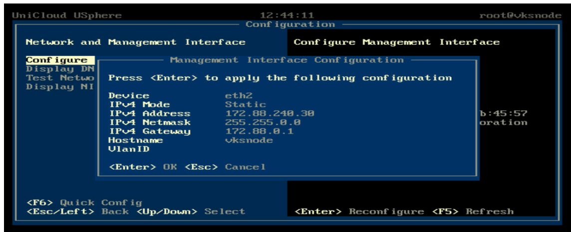
图4-29 设置静态 IP 页面
